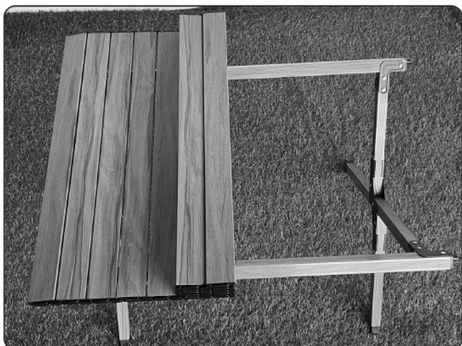
Etape 6, placez le plateau sur le cadre
